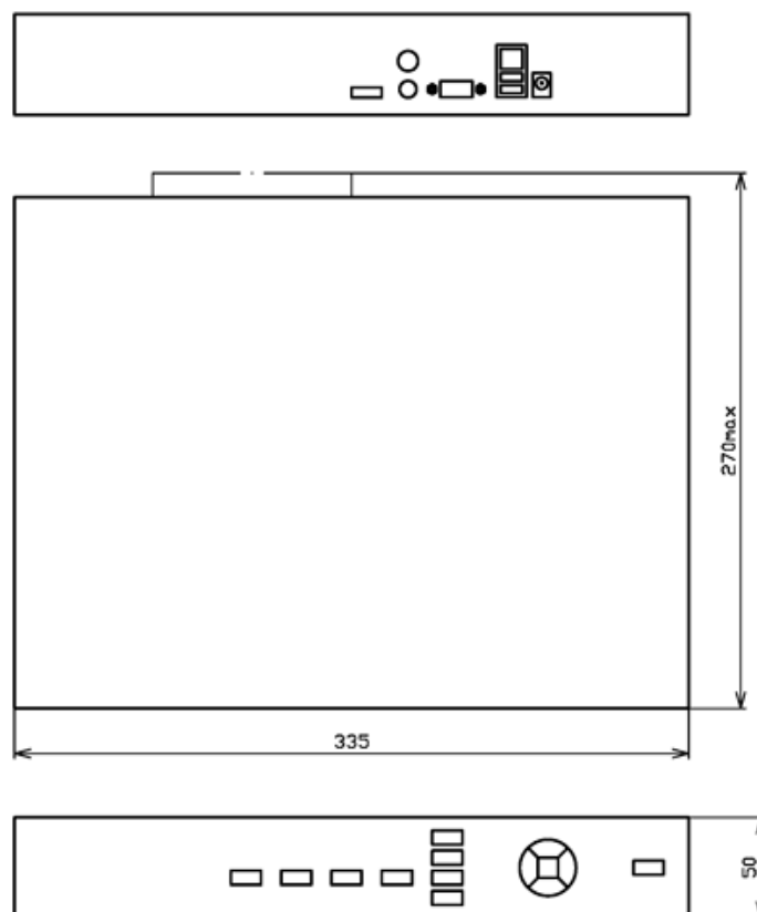
Рисунок А.21 – Габаритный чертеж видеорегистраторов ИВМС-8016, ИВМС-8032.
