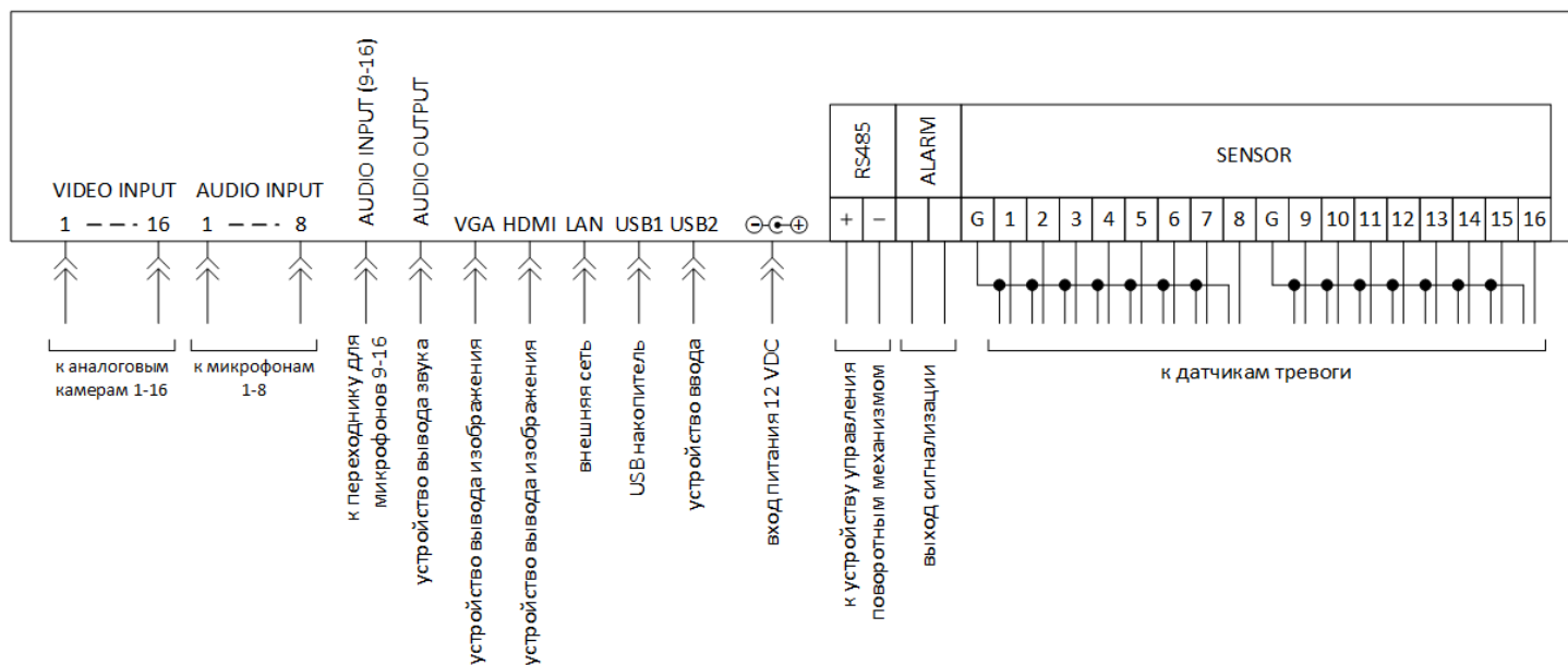
Рисунок А.8 – Схема подключения видеорегистратора ИВМ-8016.
