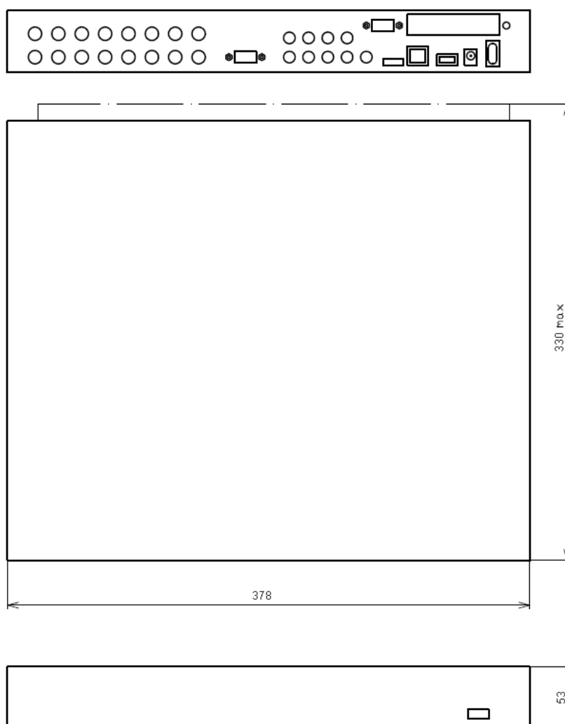
Рисунок А.9 – Габаритный чертеж ИВМ-8016.
