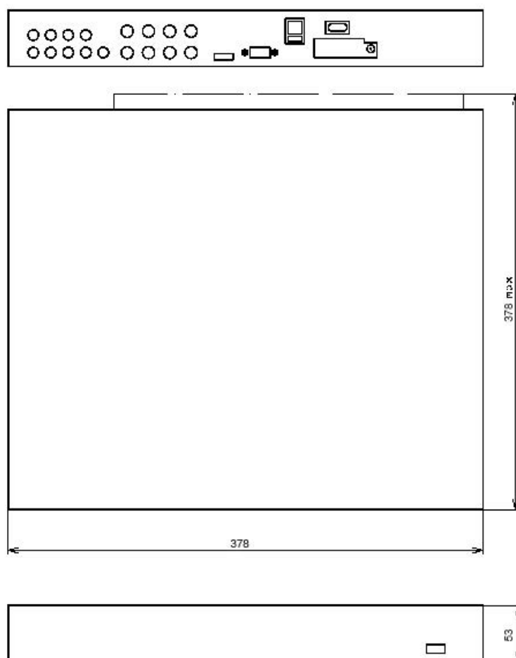
Рисунок А.6 – Габаритный чертеж ИВМ-8008.
